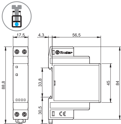
Tipo 77.01 DC Borne de jaula
